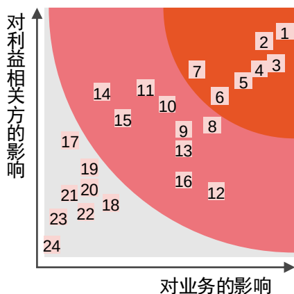
重要性矩阵
